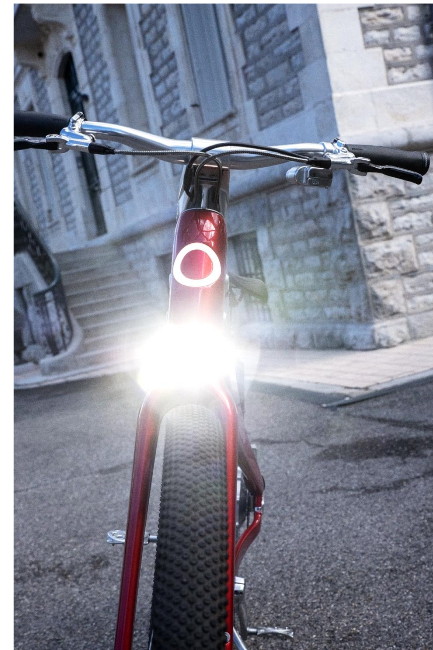
Eclairage Supernova automatique Supernova automatic light
